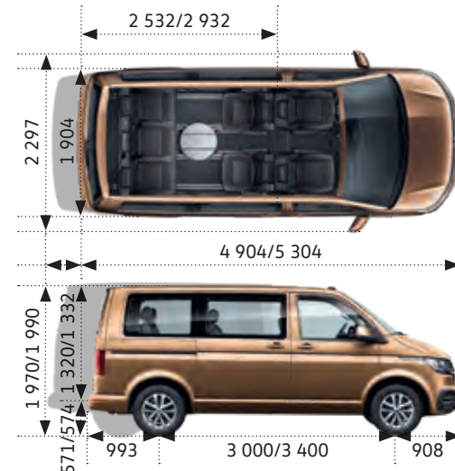
Dimensions en mm 5) (empattement court/long)
