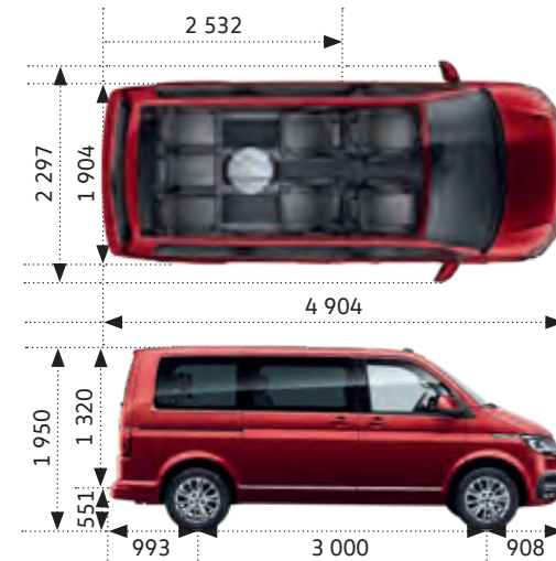
Dimensions en mm 3)
